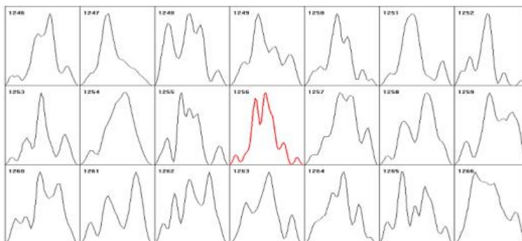
Рис.19. Ряд 0.5-минутных гистограмм, построенных по результатам измерений 3 октября 2005г. генератором
