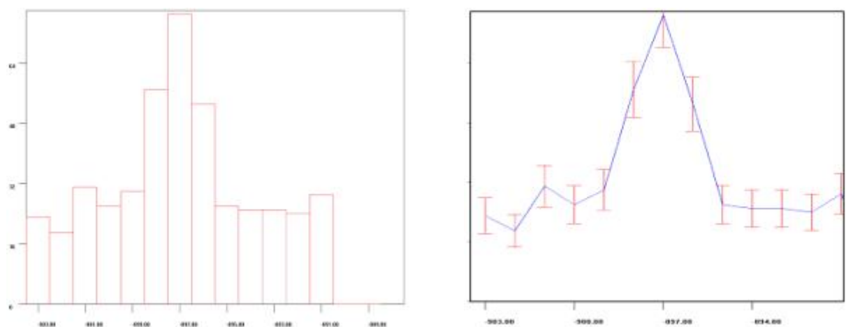
Рис. 13. Зависимость вероятности появления гистограмм сходной формы при сравнении результатов измерений 8 апреля 2005г. генератором №28 (Roger Nelson, Princeton, NJ, USA, 40,350 с.ш и 74,659 з.д.) и результатов измерений \alpha -активности ^{239}\text{Pu} в Пущино (Simon Shnoll, Puschino, Russia 54,7 с.ш., -37,6 в.д.) от величины разделяющего их интервала времени. Справа указаны среднеквадратичные ошибки. 0.5 минутные интервалы. Расчетная разность местного времени равна 449 минутам.
