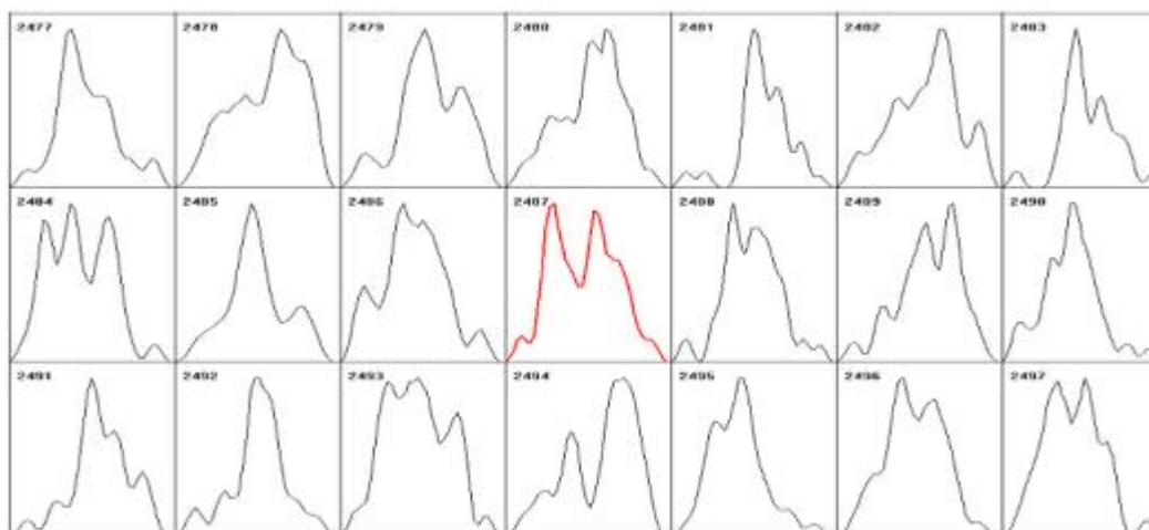
Рис.18. Ряд 0.5-минутных гистограмм, построенных по результатам измерений 8 апреля 2005г. генератором GCP №37 (John Walker, Switzerland, 47.079 с.ш. и -7.062 в.д.) Расчетный момент максимума затмения №2486, гистограмма характерной формы № 2487 отличается от расчетной на 0.5 минуты.
